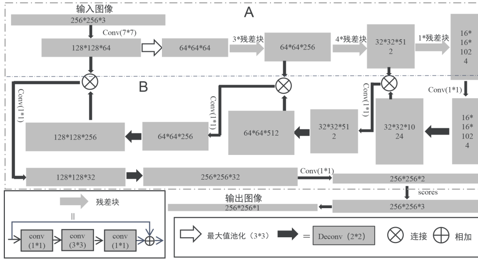
图 5 UNet 网络框架图
