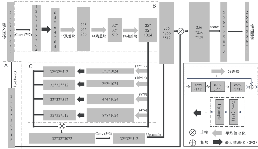
图 4 MPSPNet 网络架构图
